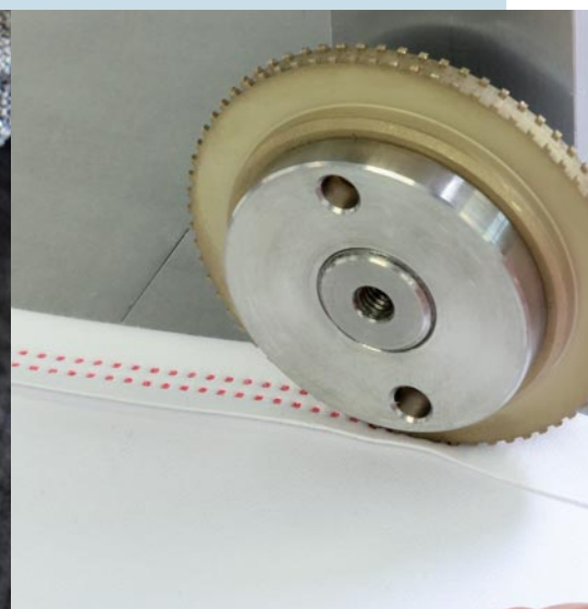
SOUDURE AUX ULTRASONS
